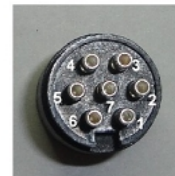
Ansicht Lötseite
